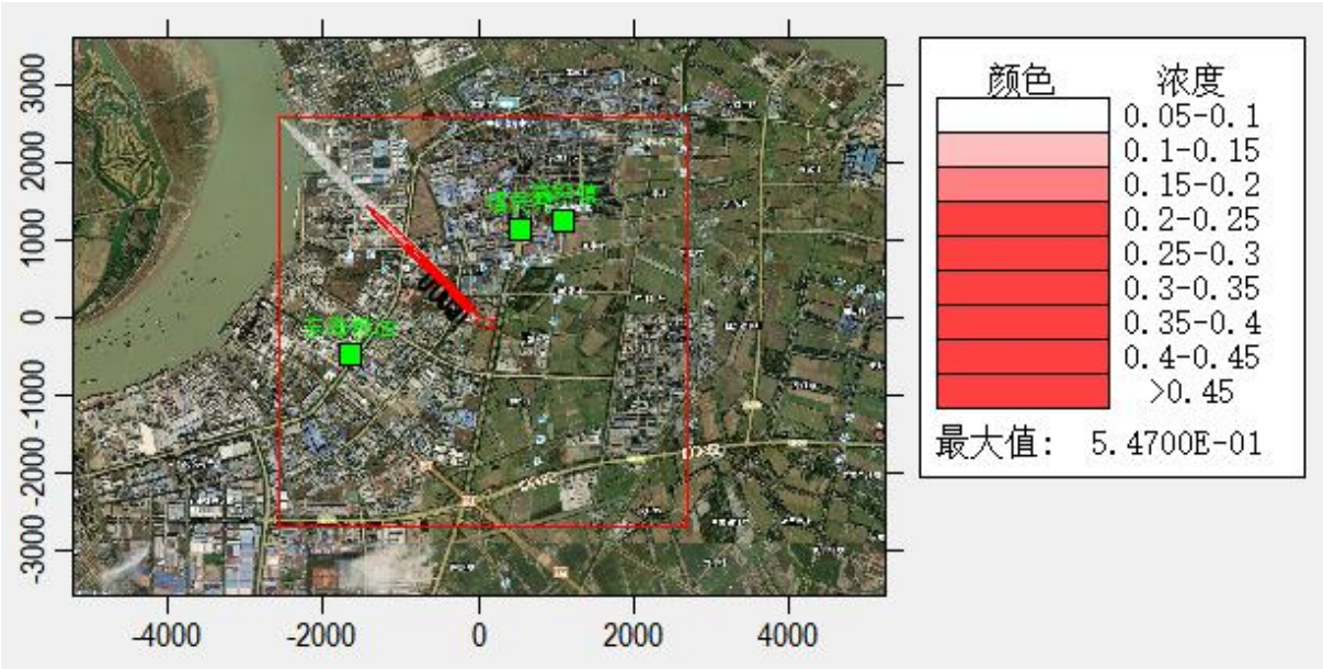
图 5.2.6.1-1 最不利气象条件下风向影响分布图
