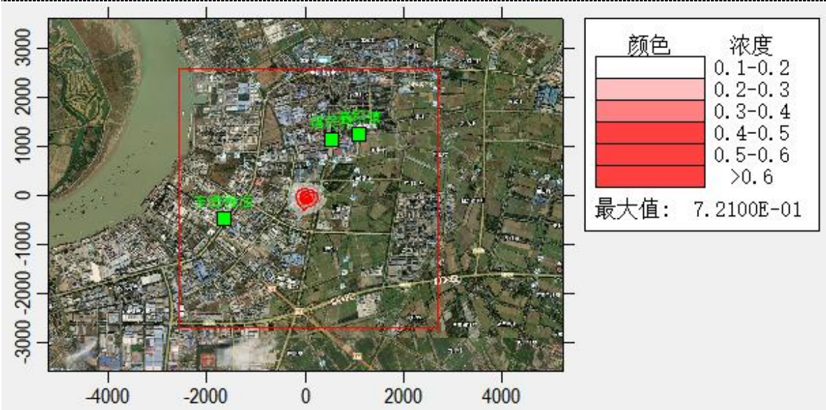
图 5.2.2.4-4 非甲烷总烃小时浓度贡献分布图
