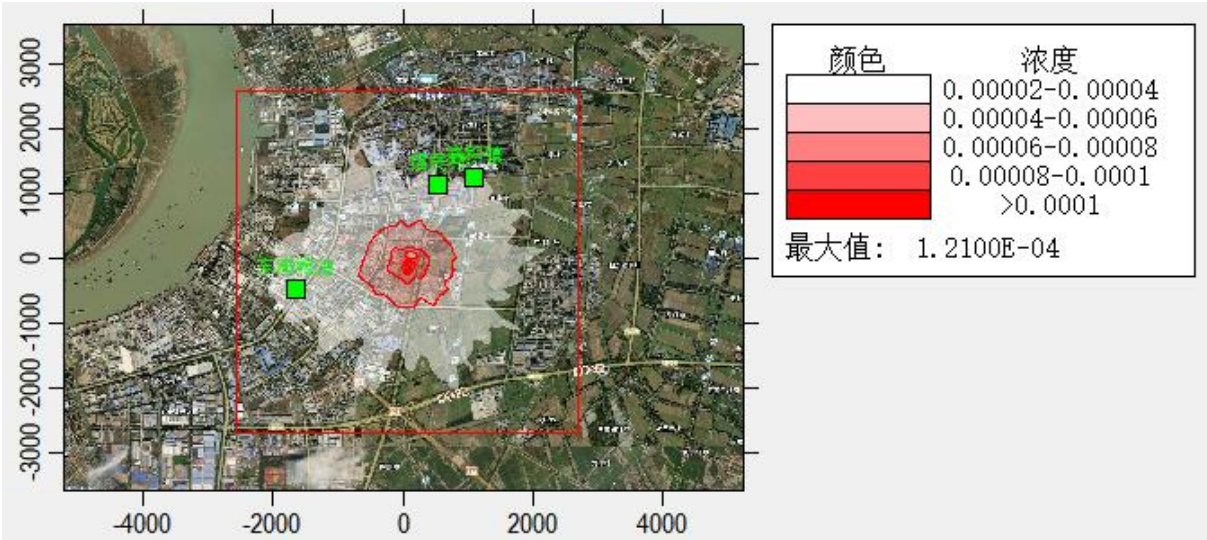
图 5.2.2.4-1 颗粒物小时浓度贡献分布图
