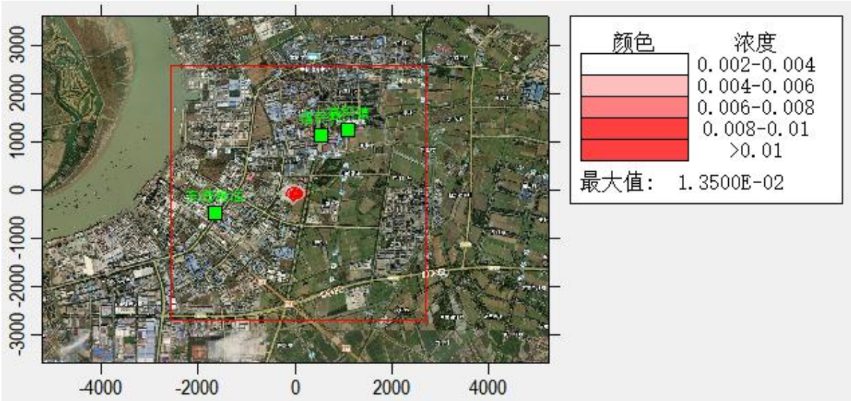
图 5.2.2.4-6 非甲烷总烃年均浓度贡献分布图
