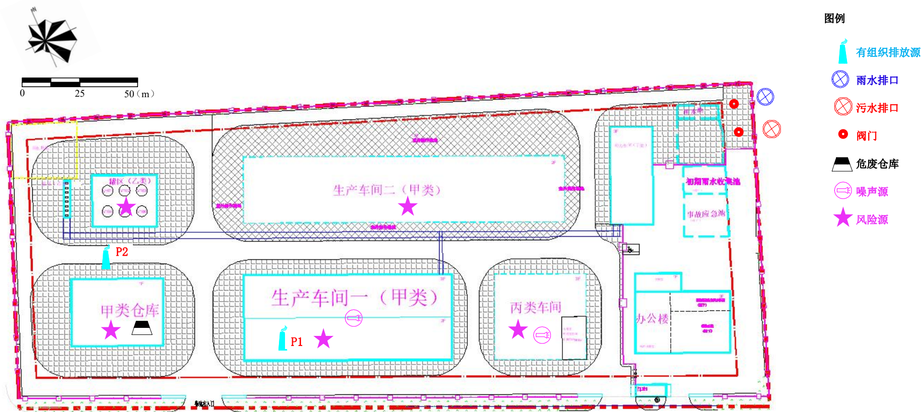
图 3.1.3-1 厂区平面布置图
