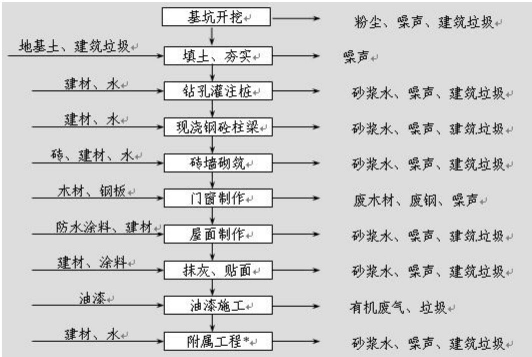
图 3.3.1-1 施工期建筑工艺流程图
