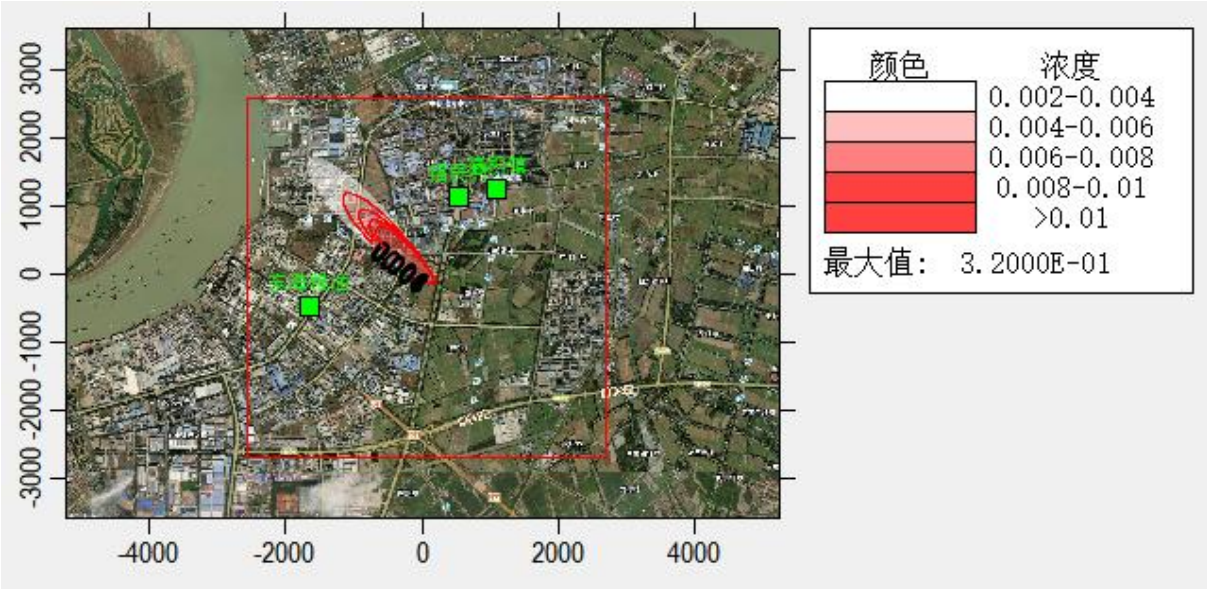
图 5.2.6.1-1 最常见气象条件下风向影响分布图
