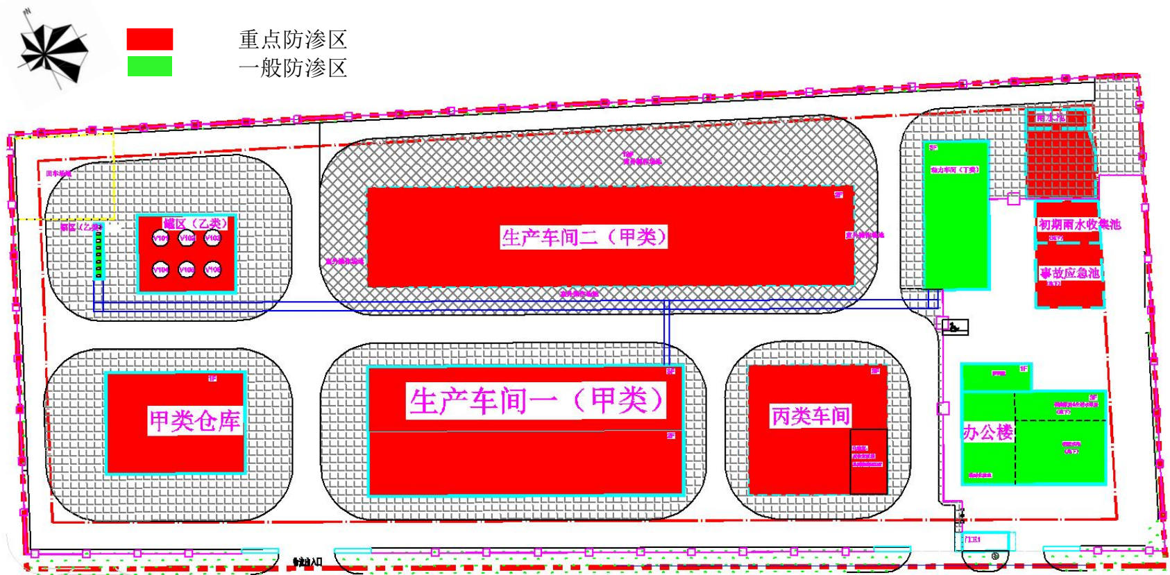
图 6.5-1 厂区分区防渗图
