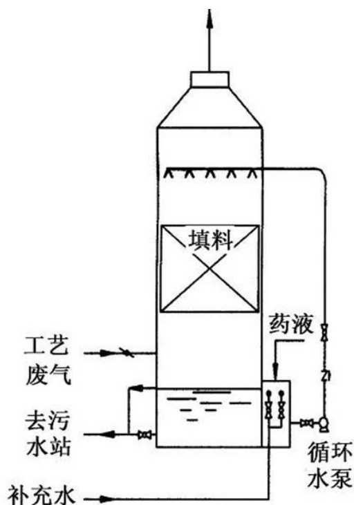
图 6.1.1.2-1 水喷淋塔示意图
