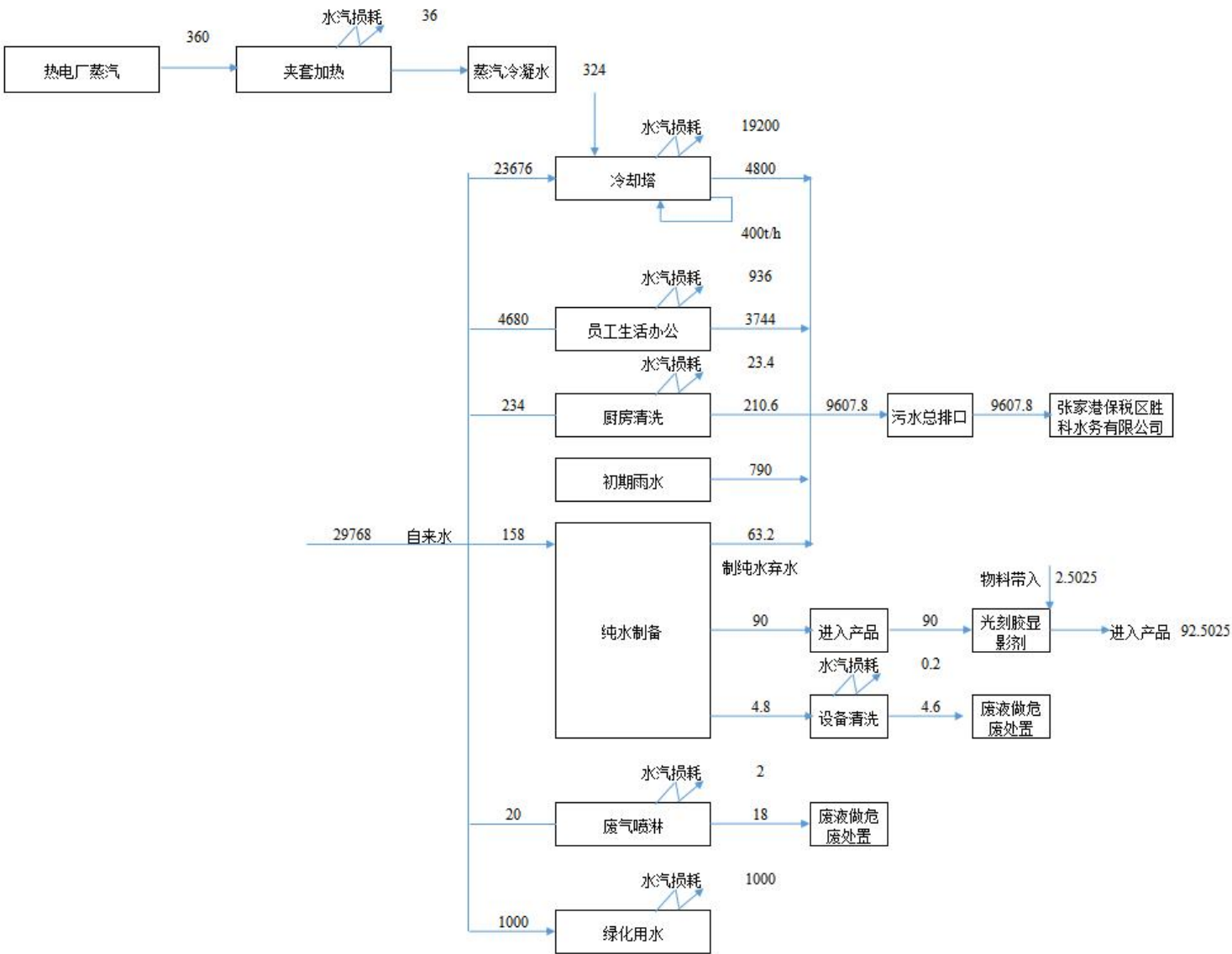
图 3.2.6-1 本项目水平衡图（单位：t/a）
