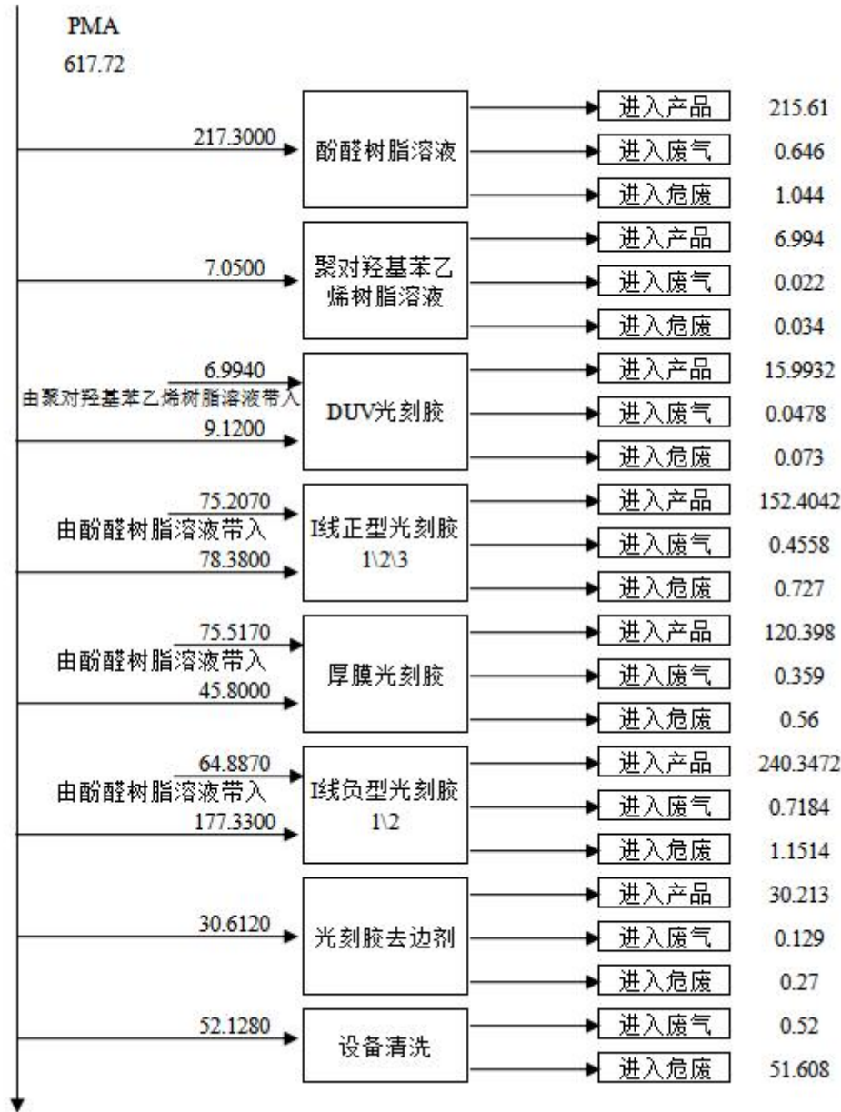
图 3.3.7-1 PMA 溶剂平衡图 (单位: t/a)
