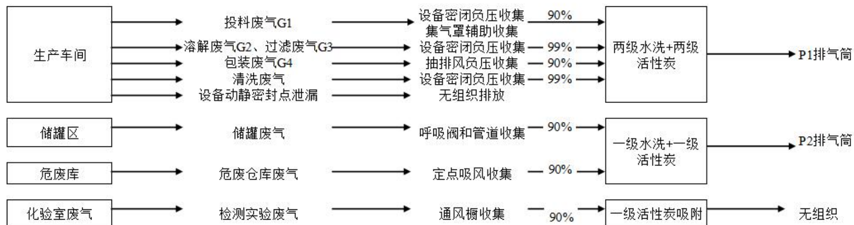
图 6.1.1.1-1 废气收集及处理示意图
