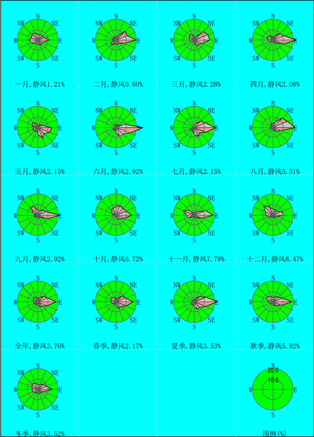
图 5.2.1-4 张家港 2021 年风频玫瑰图
